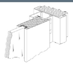
CERCO ENRASADO EMBOCADURAS
